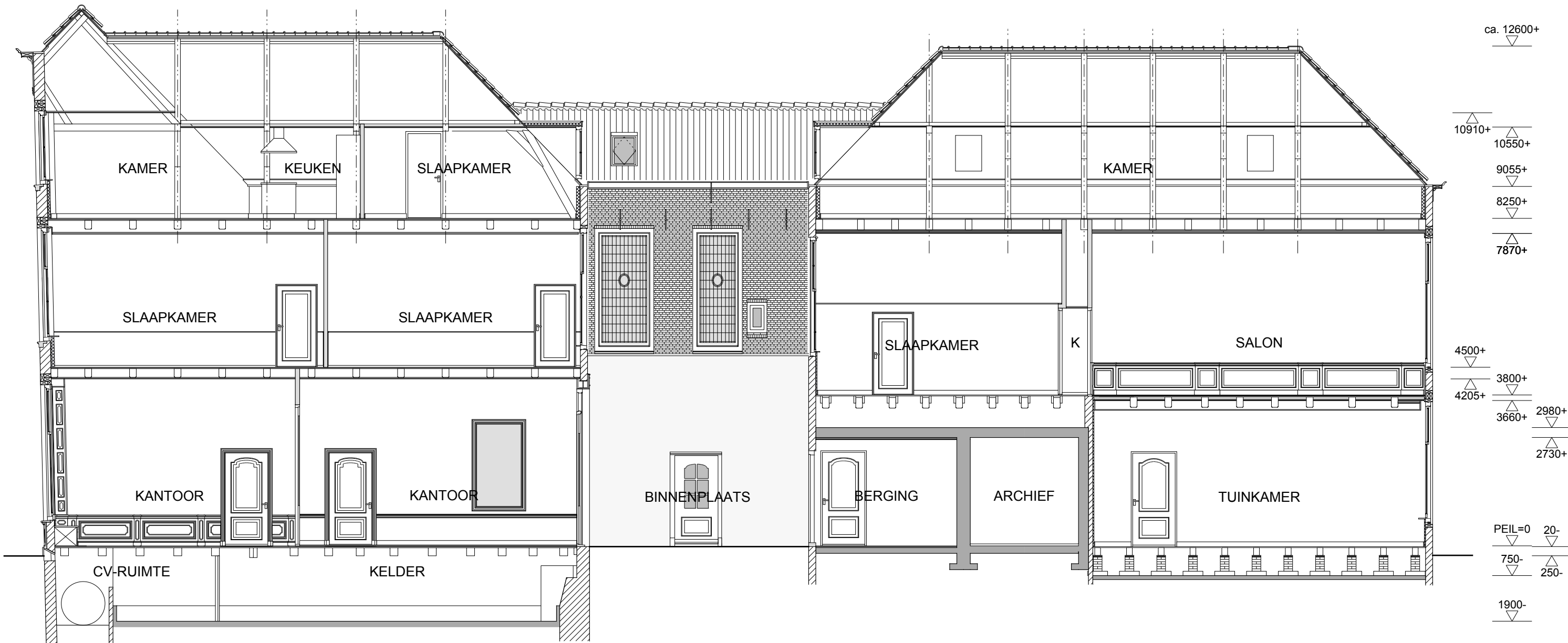
DOORSNEDE A-A'
