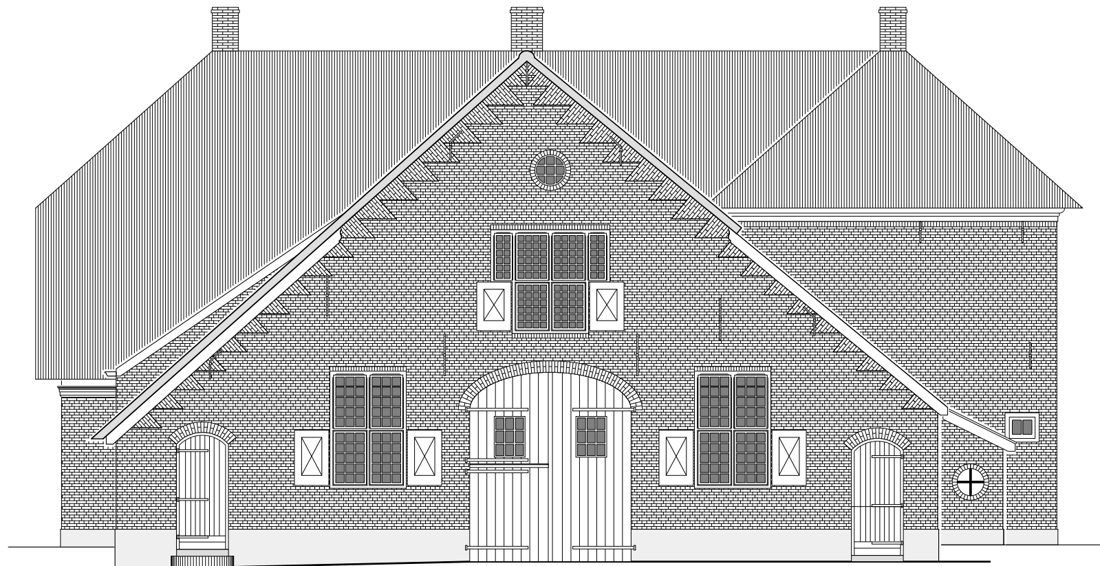
ACHTERGEVEL
